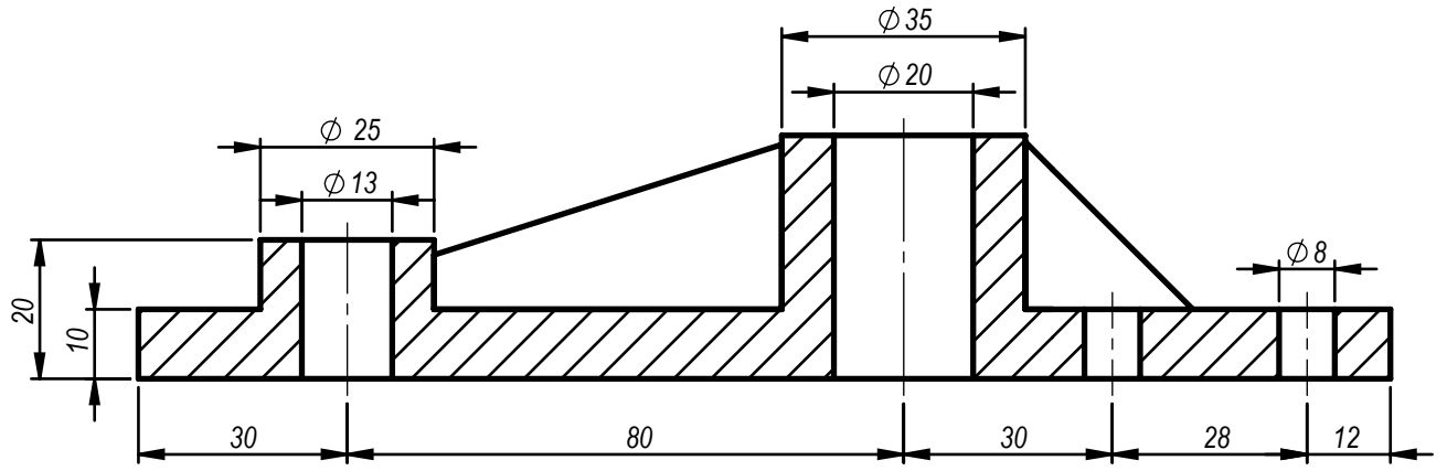
SECTION A-A SCALE 1 : 1.2
